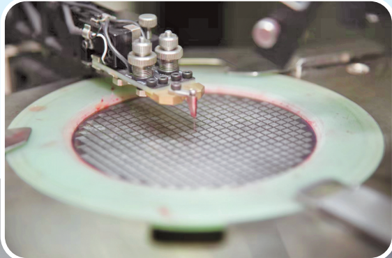
划片室内，探针检测硅片上的芯片是否正常。
